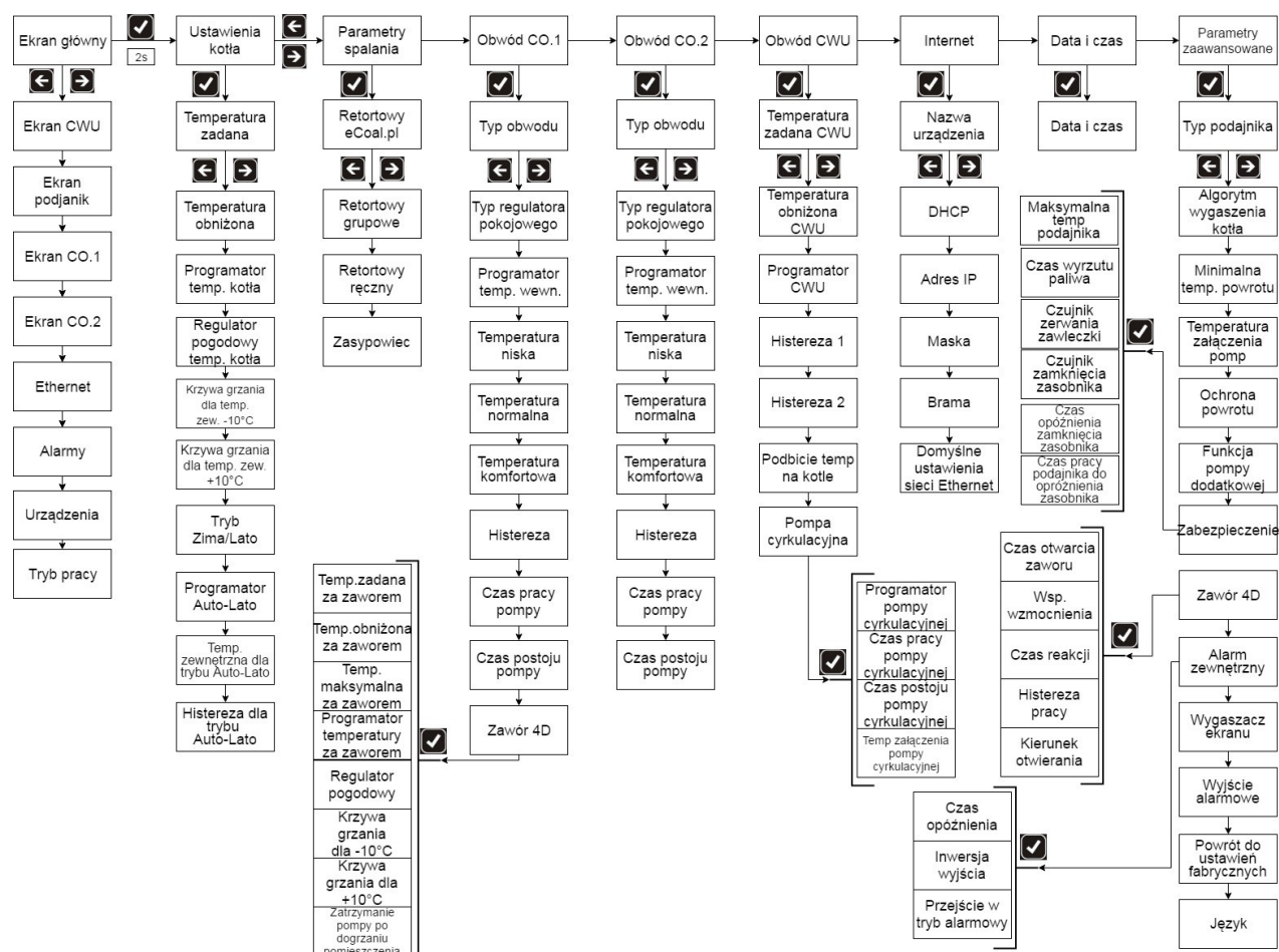
Ilustracja 17: Schemat menu sterownika
