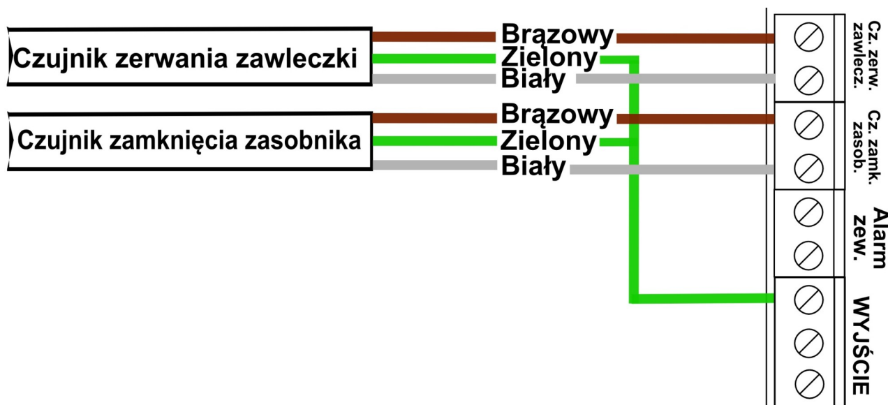
Ilustracja 4: Podłączenie czujników: zerwania zawleczki oraz zamknięcia zasobnika
